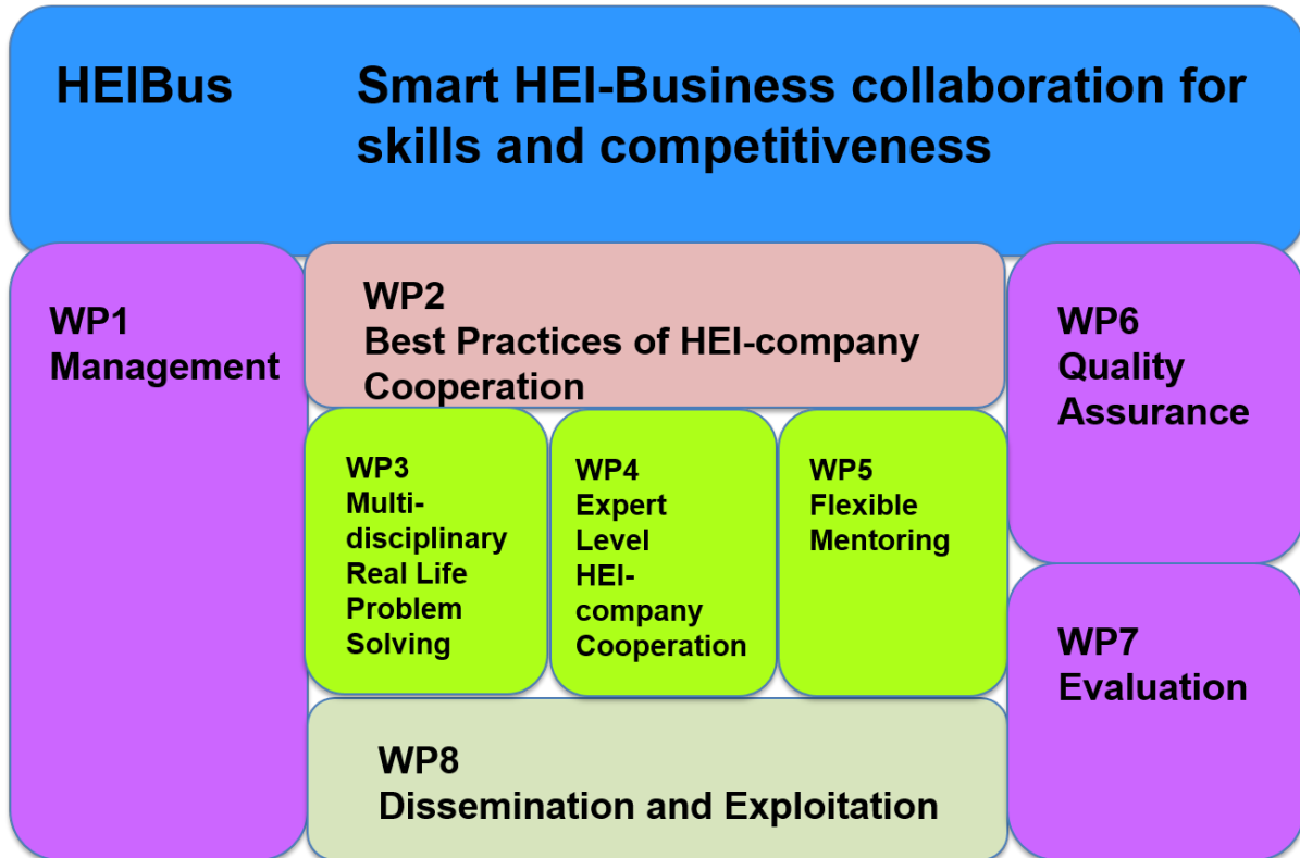
Kuva 2. HEIBus-projektin työpaketit
